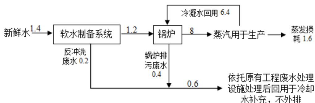
图 2-1 技改项目水平衡图( \text{m}^3/\text{d} )
